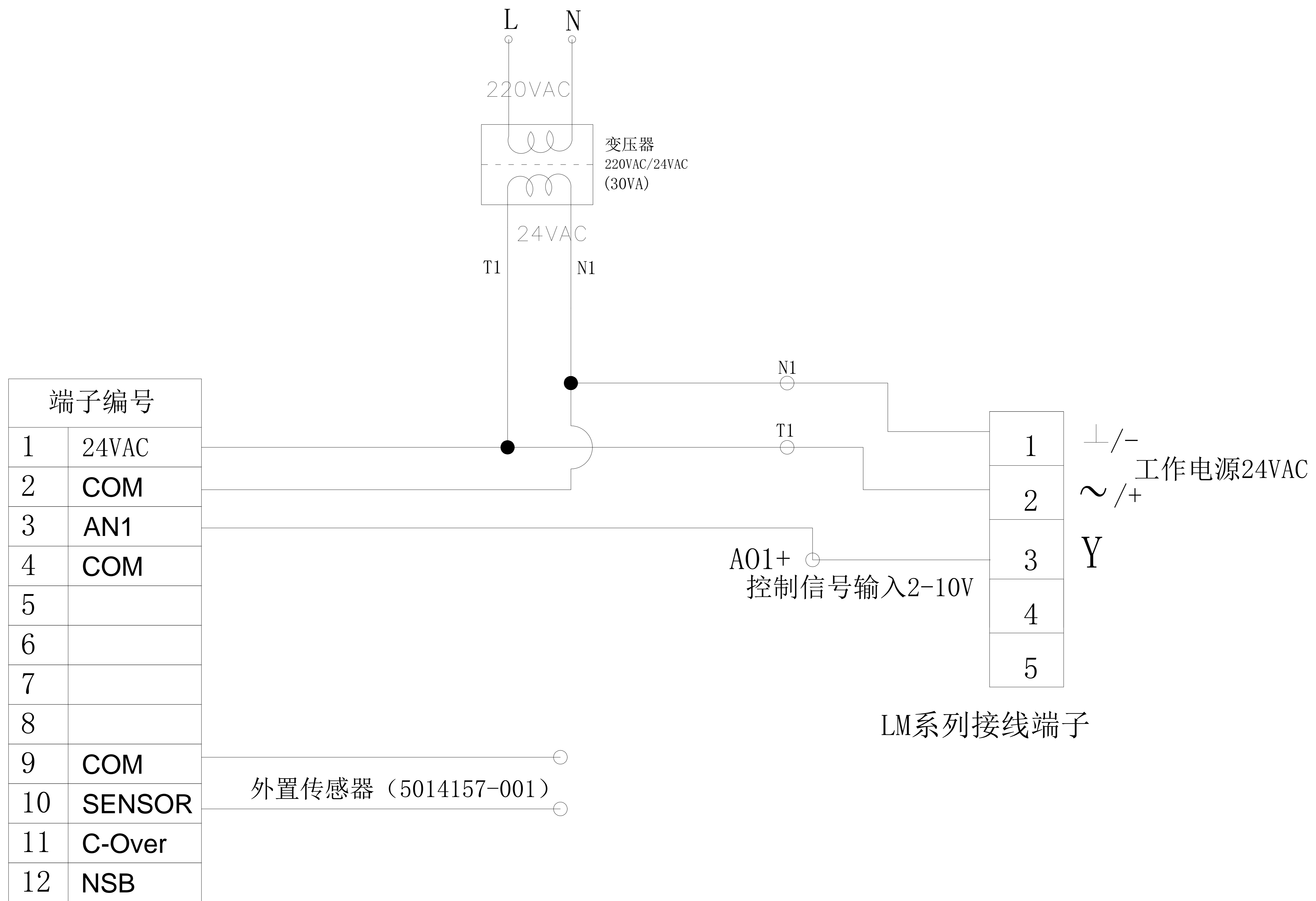
TB7980接线端子
