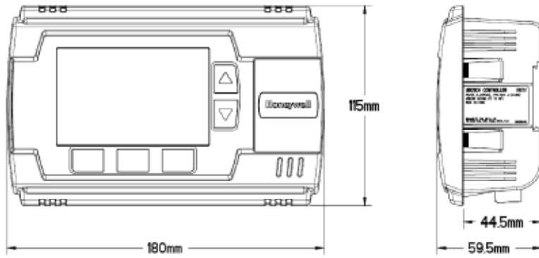
图1 产品尺寸
